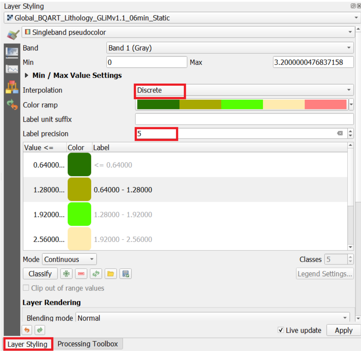
Fig. 2: Layer Styling
